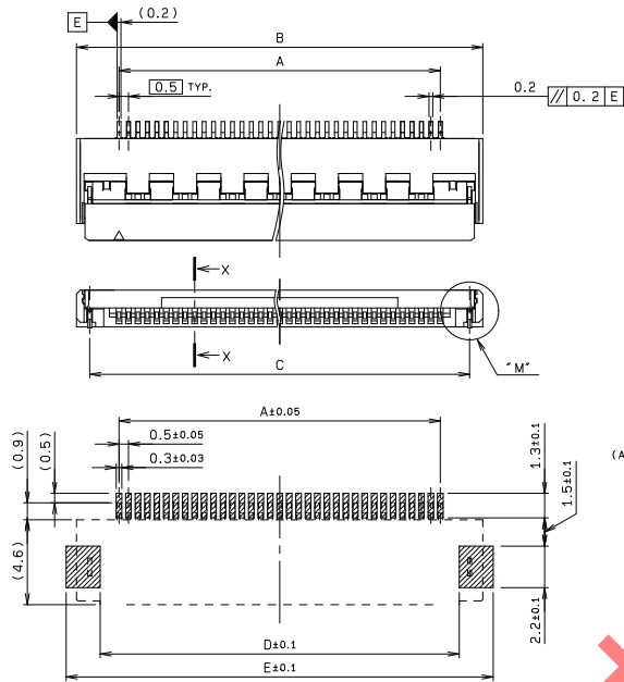
推奨基板取付け寸法 MOUNTING LAYOUT
