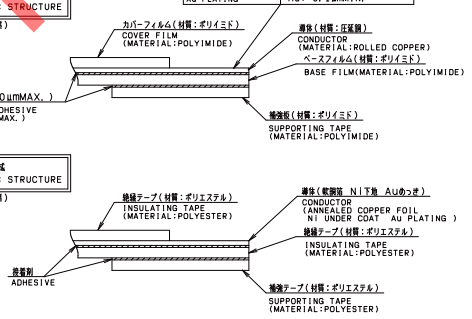
FPC構成 FPC STRUCTURE (縦横仕様)
