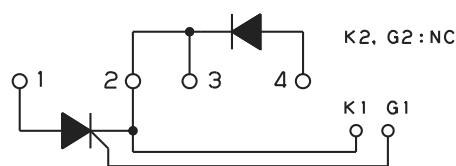
回路構成 Circuit Schema
