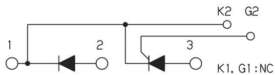
回路構成 Circuit Schema
