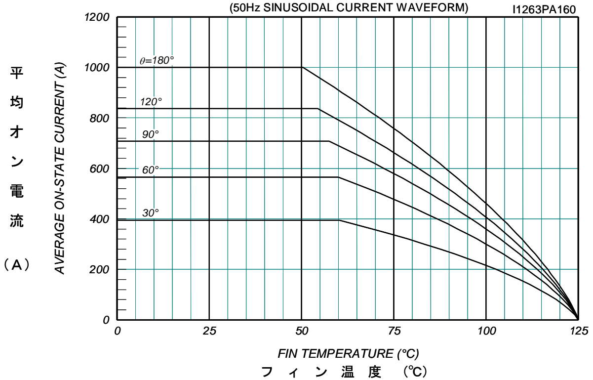
平均オン電流 - フィン温度定格 AVERAGE ON-STATE CURRENT VS. FIN TEMPERATURE
