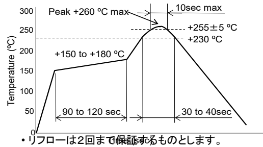
図5 推奨リフロープロファイル(鉛フリー半田対応)
