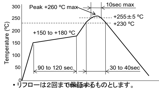
図5 推奨リフロープロファイル(鉛フリー半田対応)
