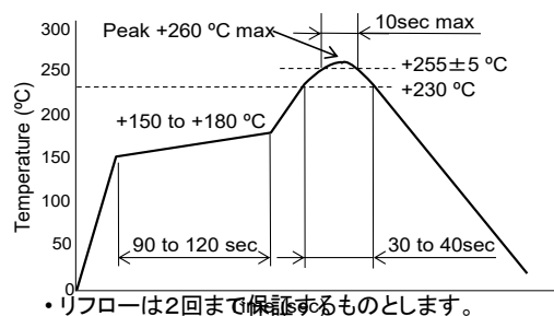
図5 推奨リフロープロフィール(鉛フリー半田対応)
