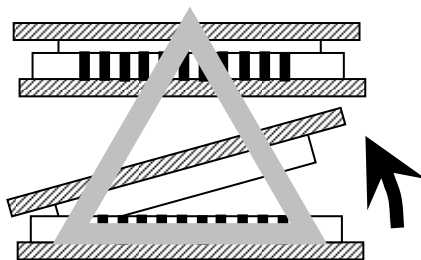
長手方向 (△)
