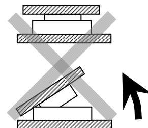
短手方向 (×)
