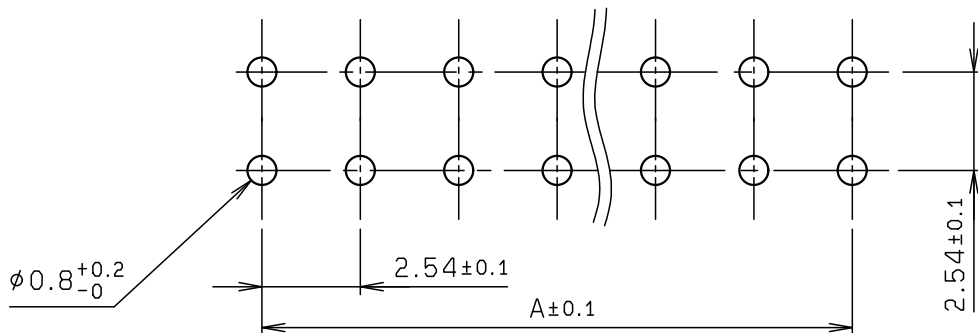
基板穴明け寸法 MOUNTING LAYOUT
