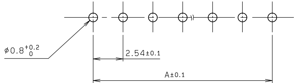
基板穴明け寸法図 MOUNTUNG LAYOUT
