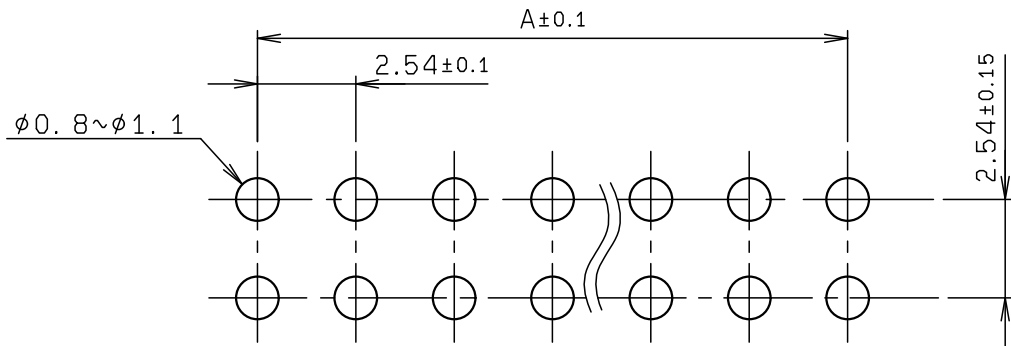
基板取付け寸法図 MOUNTING LAYOUT
