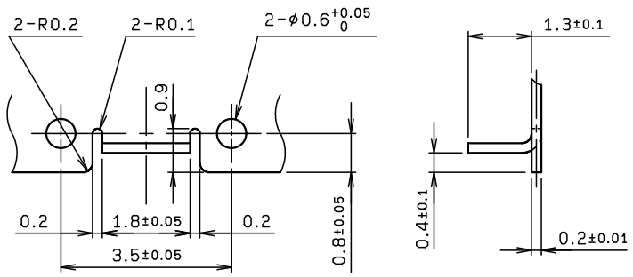
シールドケース形状 SHIELDING CASE FORM
