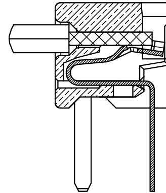
嵌合断面図 MATED STATE
