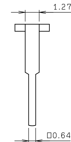
コンタクトテール詳細図 CONTACT TAIL (S=5:1)
