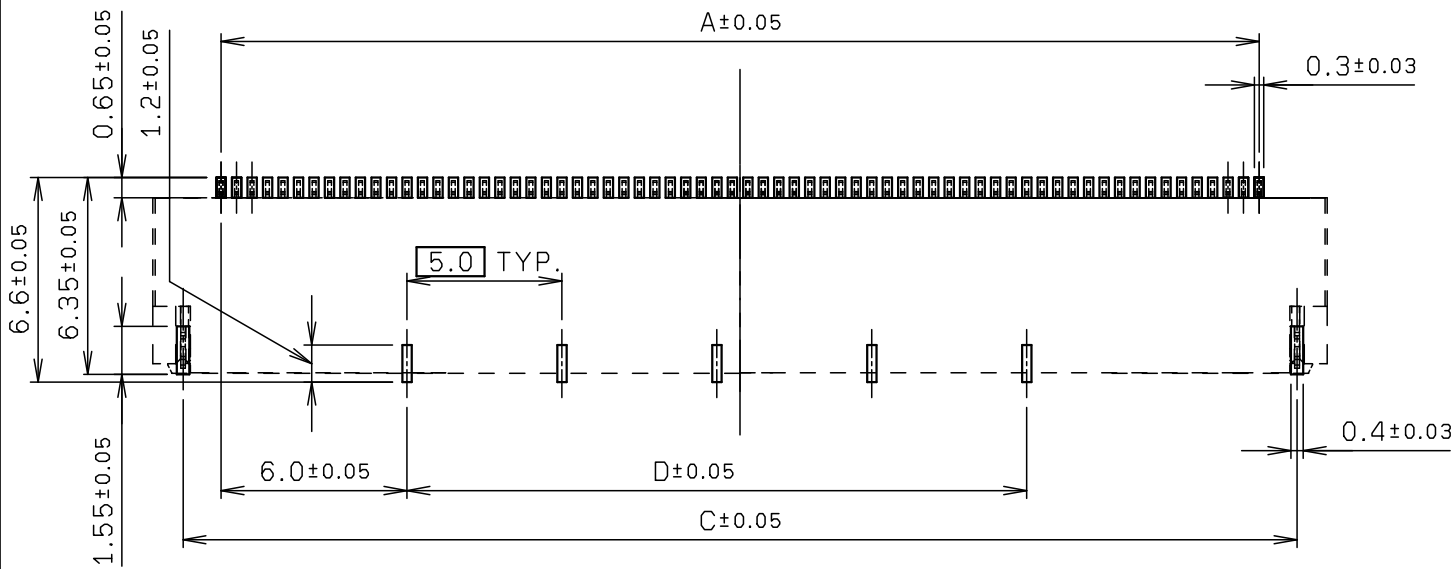
推奨パターン寸法 RECOMMENDED PATTERN LAYOUT
