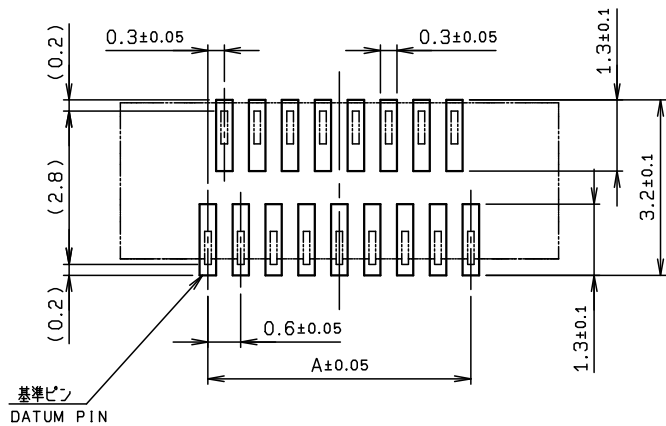
推奨パターン寸法 (コネクタ搭載側) RECOMMENDED PATTERN LAYOUT
