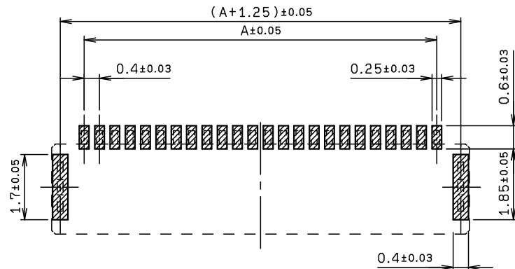
基板取付け寸法 MOUNTING LAYOUT
