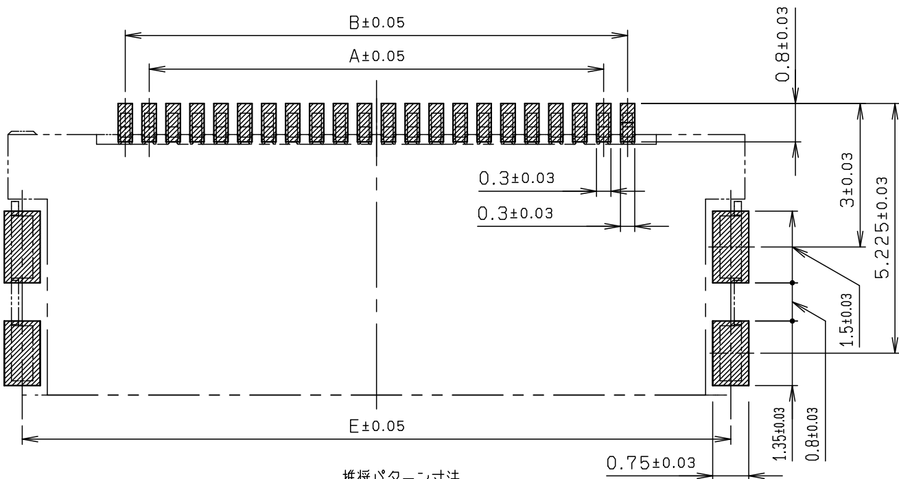
推奨パターン寸法 RECOMMENDED PATTERN LAYOUT
