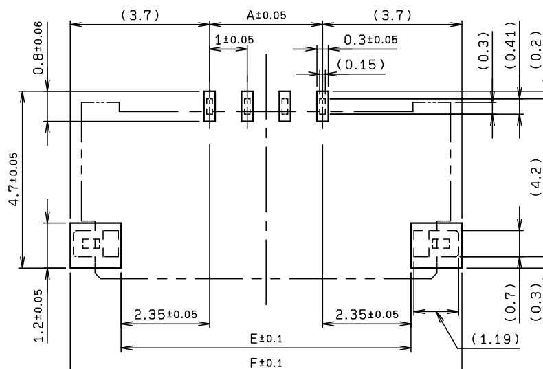
参考パターン寸法 REFERENCE PATTERN LAYOUT
