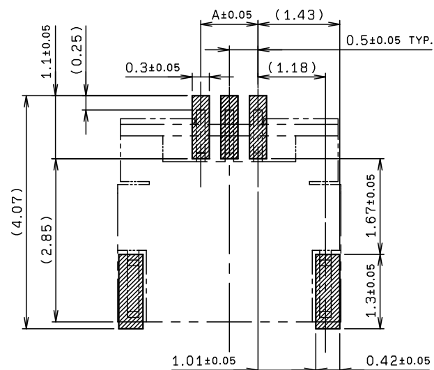
推奨基板取付け寸法 MOUNTING LAYOUT
