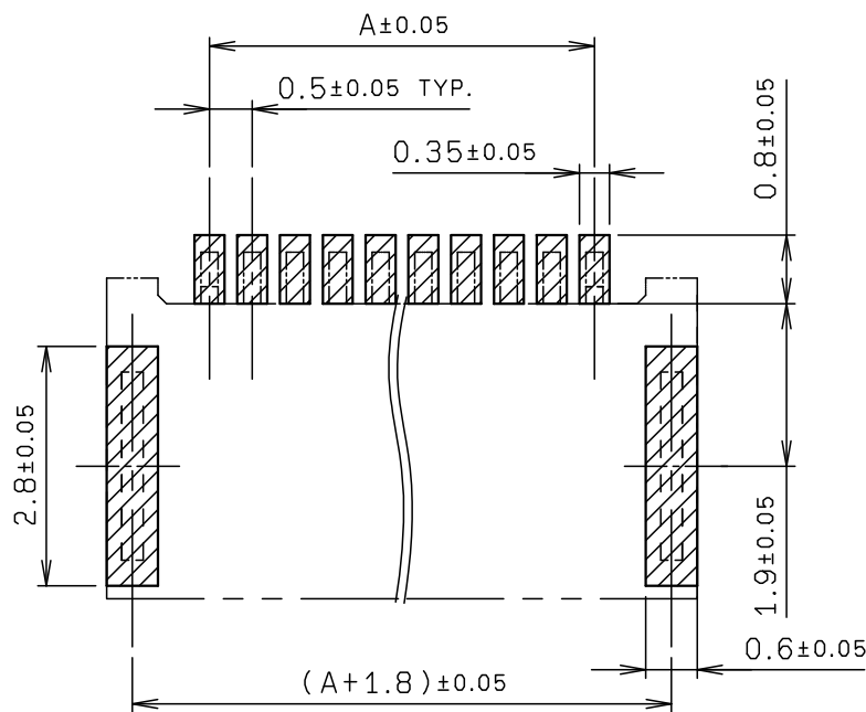
基板取付け寸法 MOUNTING LAYOUT
