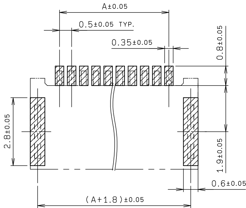
基板取付け寸法 MOUNTING LAYOUT
