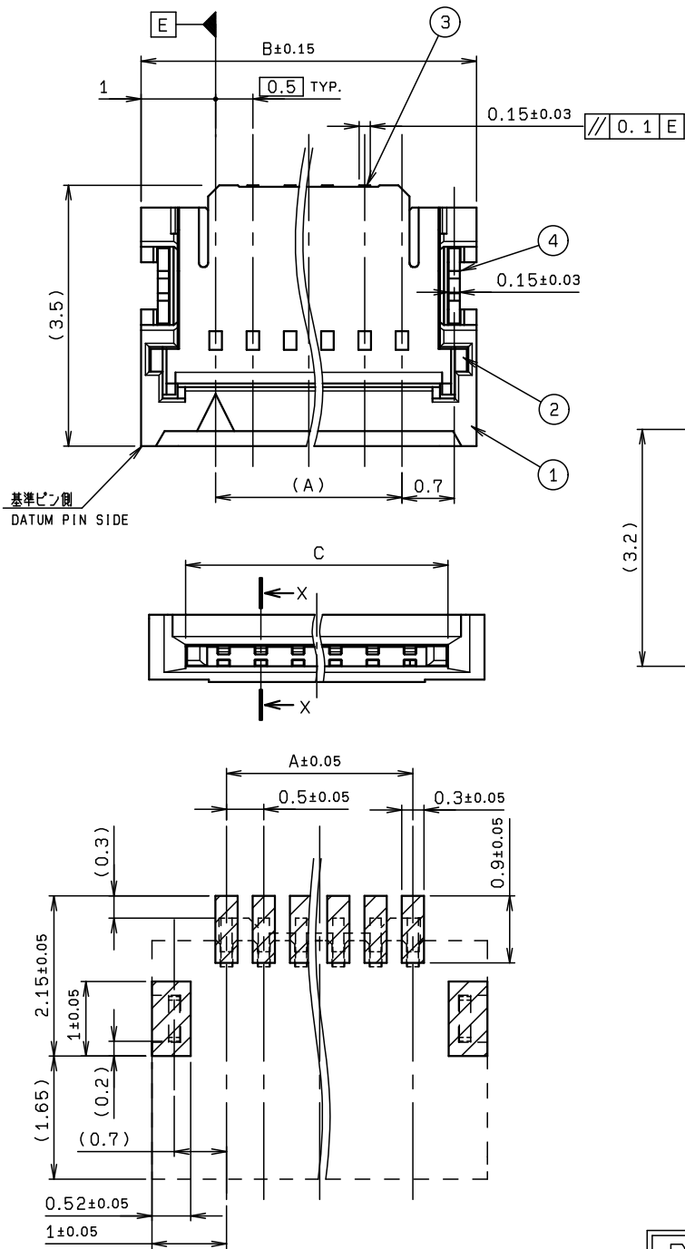
推奨基板取付け寸法 MOUNTING LAYOUT
