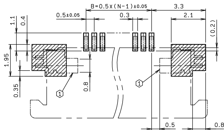
推奨基板取付寸法（コネクタ搭載側）
