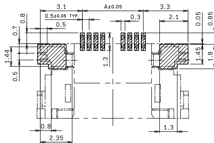
基板取付け寸法 MOUNTING LAYOUT
