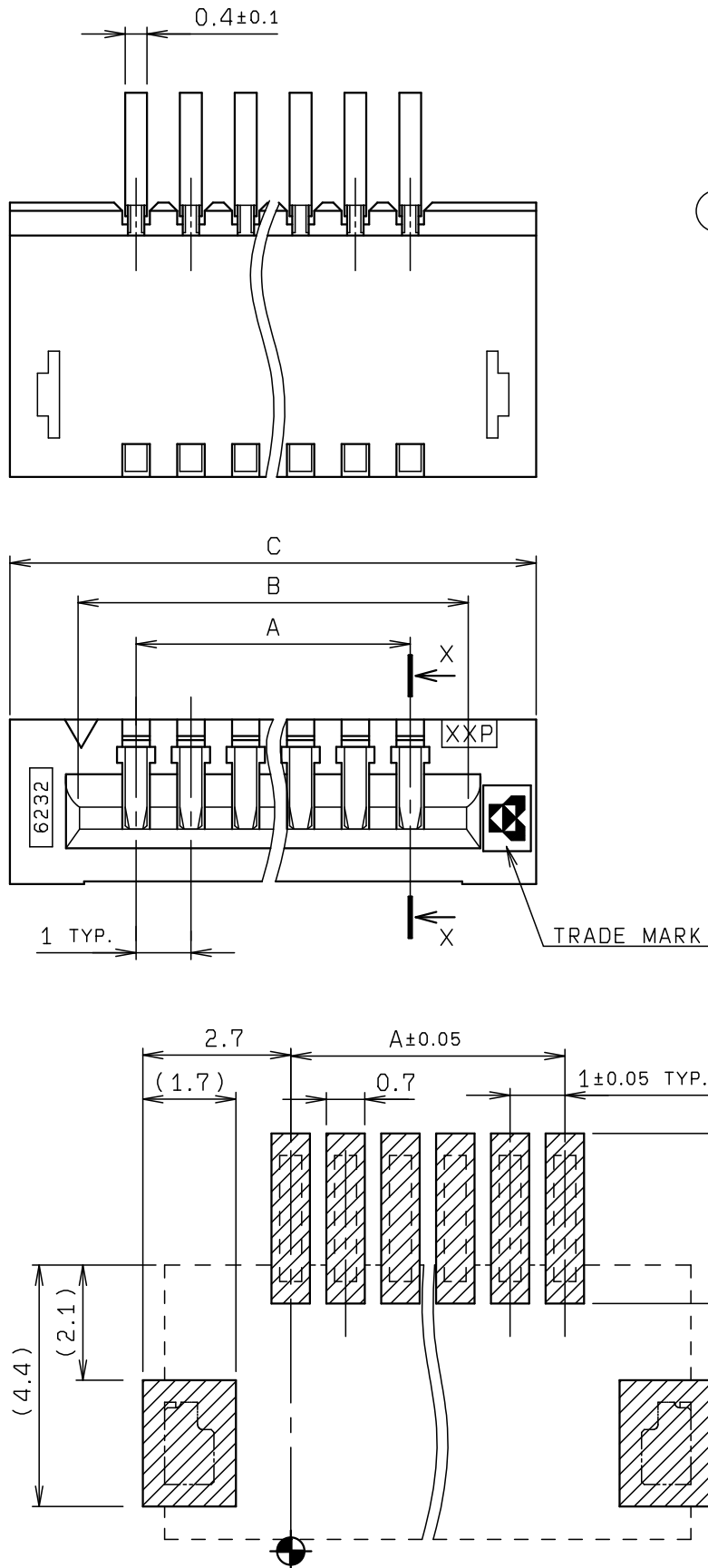
基板取付け寸法 (コネクタ搭載側) MONTING LAYOUT (CONN. MOUNTING SIDE)
