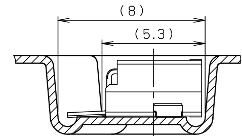
上接点タイプ UPPER CONTACT TYPE コネクタ型番: 00 6232 1XX 103 800 + CONTACT P/N
