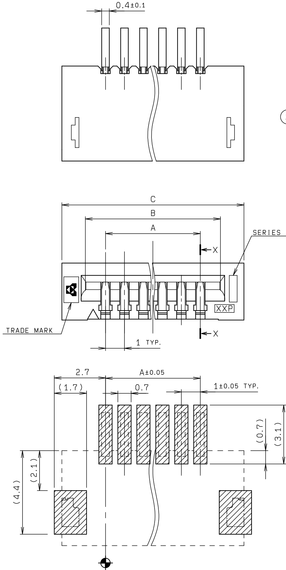
基板取付け寸法（コネクタ搭載側） MONTING LAYOUT (CONN. MOUNTING SIDE)
