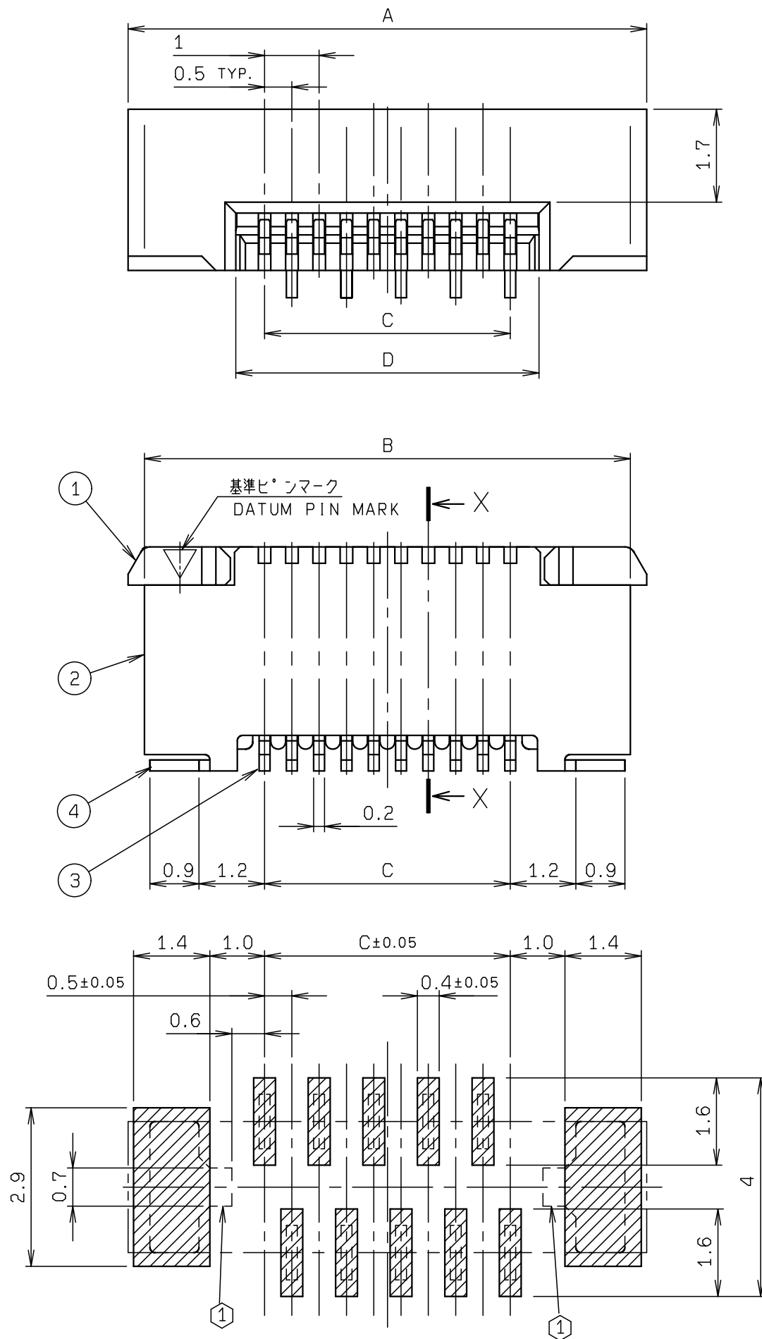
推奨基板取付寸法 (コネクタ搭載側) MOUNTING LAYOUT (CONN. MOUNTING SIDE)
