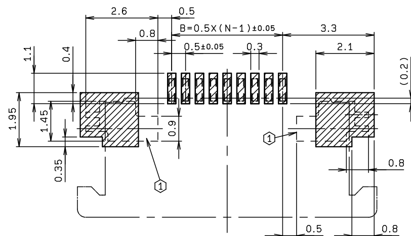
基板取付寸法 MOUNTING LAYOUT
