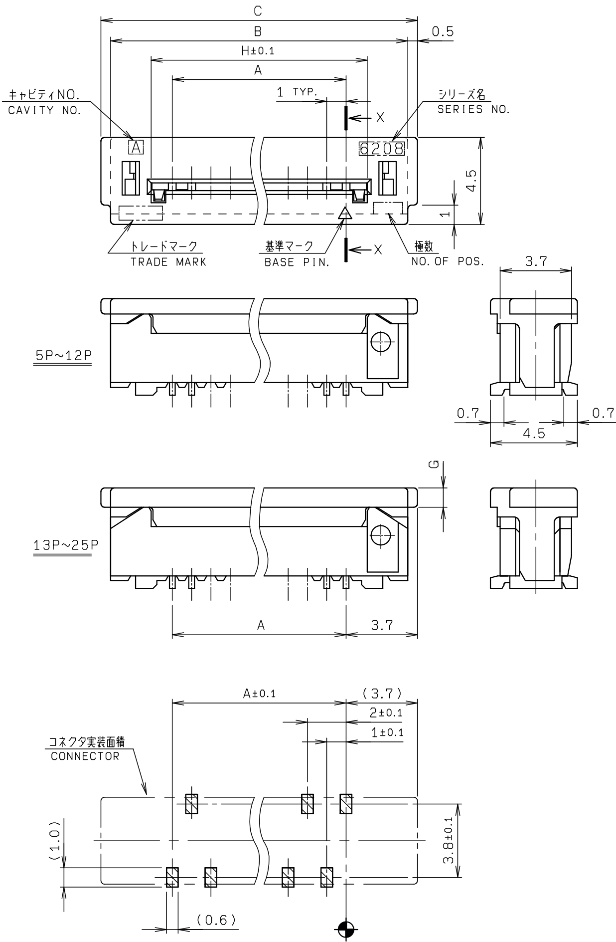
基板取付寸法 MOUNTING LAYOUT
