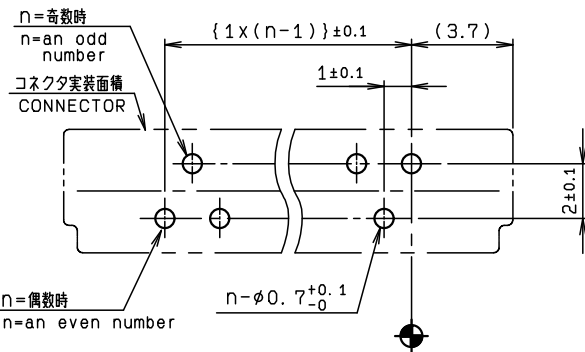
基板取付寸法 (コネクタ搭載側) MOUNTING LAYOUT t=1.2~1.6 mm
