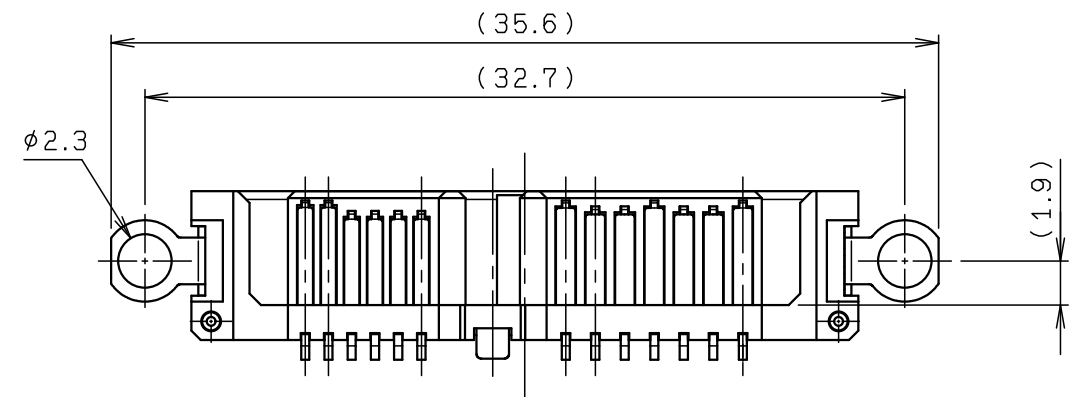
ANCHOR VARIATION P/N 10 XXXX 013 002 XXX +
