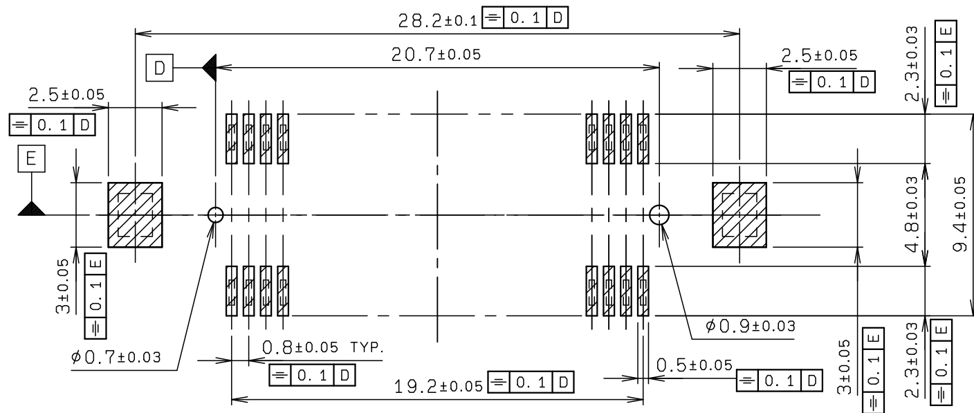
基板取り付け寸法 MOUNTING LAYOUT
