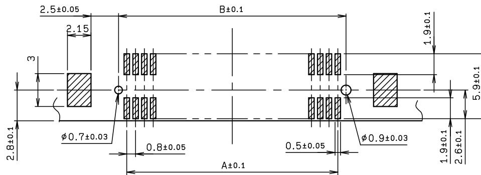
基板取付寸法 MOUNTING LAYOUT
