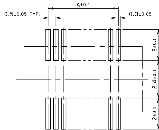
基板取付け寸法 MOUNTING LAYOUT
