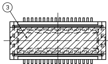
吸着テープ位置 POSITION OF VACUUM TAPE
