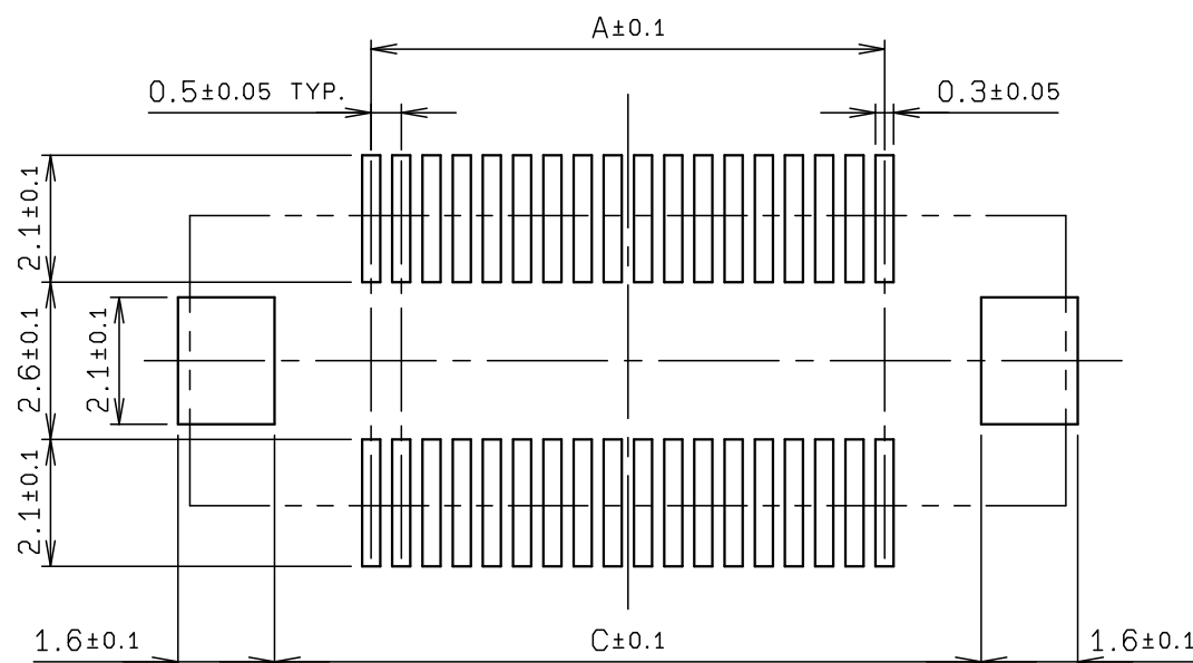
基板取付け寸法 RECOMMENDED LAYOUT
