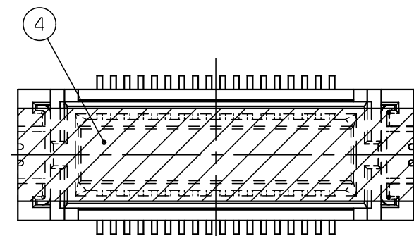
吸着テープ位置 POSITION OF VACUUM TAPE
