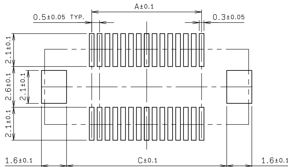
推奨基板取付け寸法 MOUNTING LAYOUT
