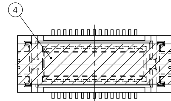
吸着テープ位置 POSITION OF VACUUM TAPE
