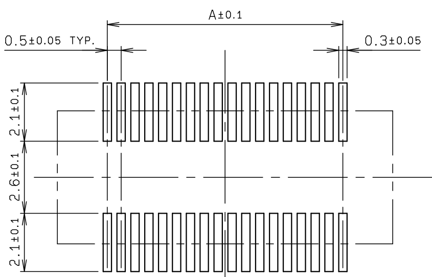
基板取り付け寸法 MOUNTING LAYOUT
