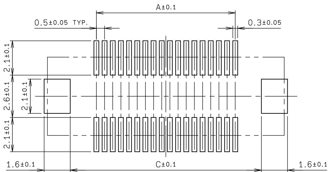
基板取り付け寸法 RECOMMENDED LAYOUT
