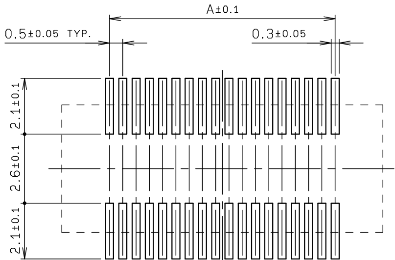
基板取付け寸法 MOUNTING LAYOUT
