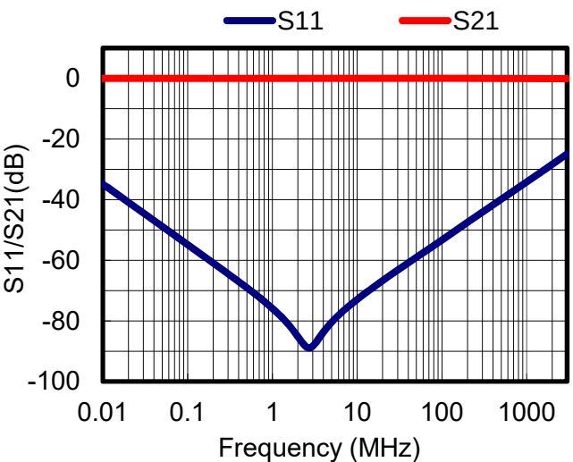
S parameters(Series)
