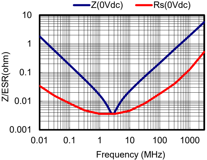
Impedance/ESR
