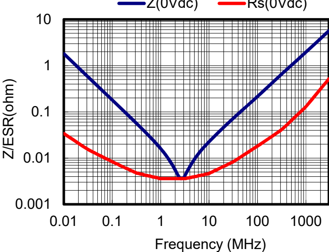
Impedance/ESR
