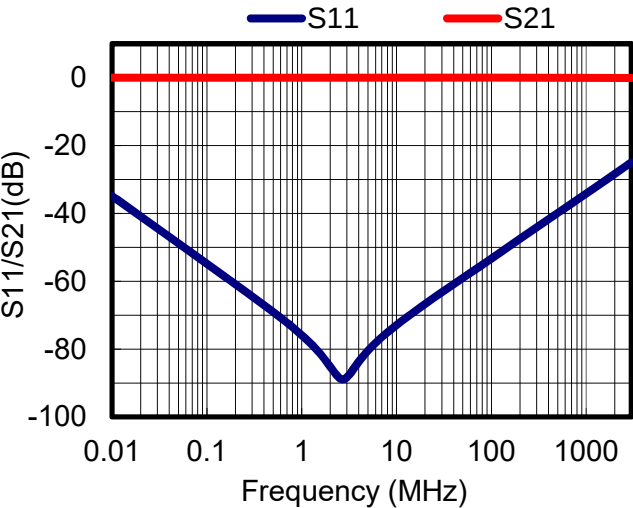
S parameters(Series)
