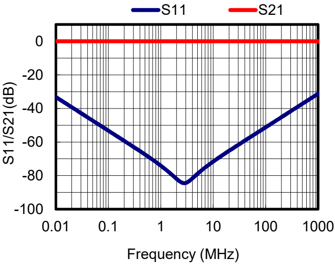
S parameters(Series)
