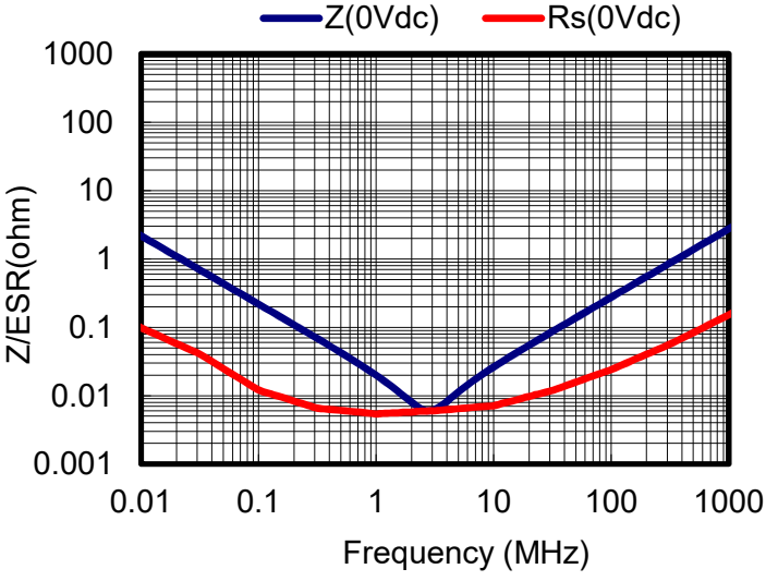
Impedance/ESR
