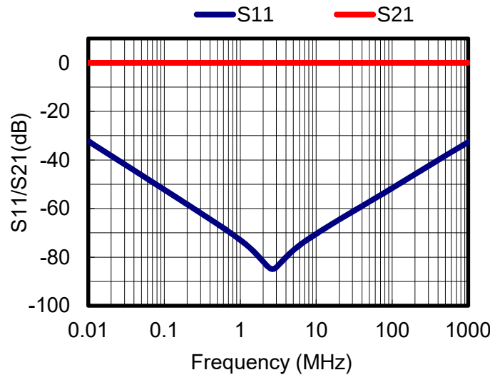
S parameters(Series)
