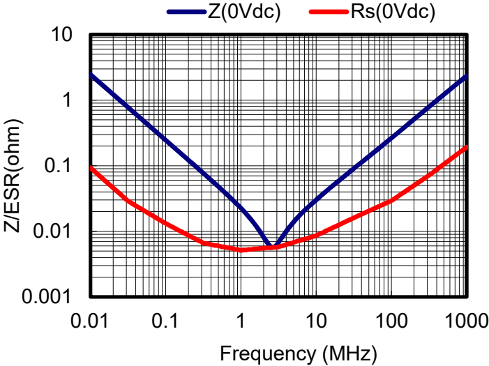
Impedance/ESR
