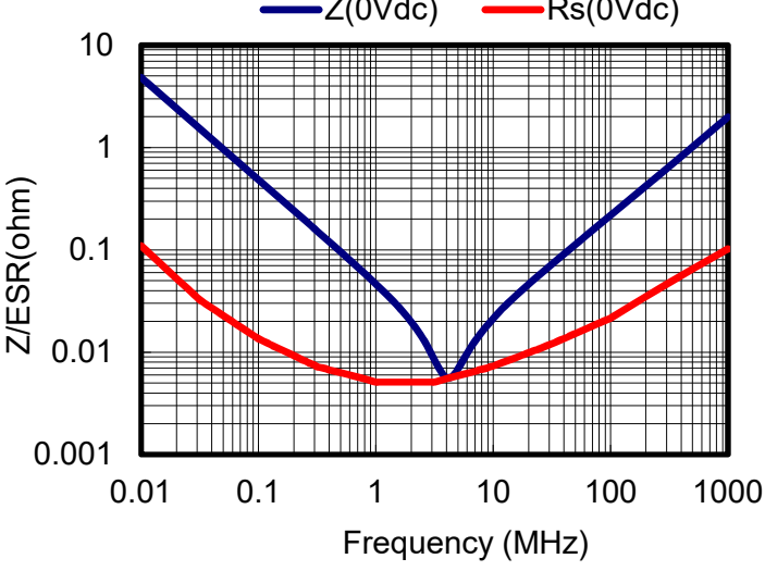
Impedance/ESR
