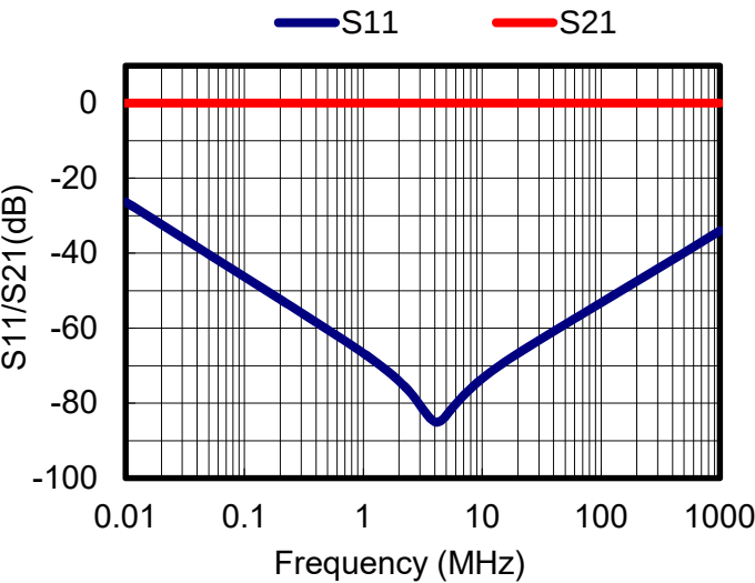
S parameters(Series)
