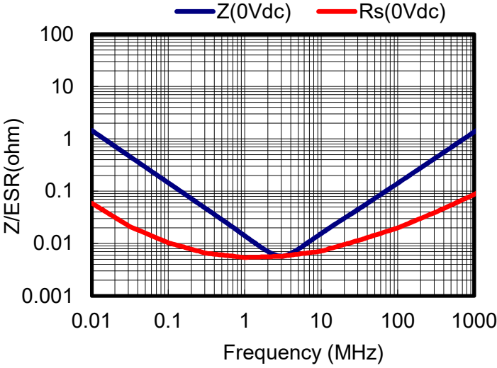
Impedance/ESR
