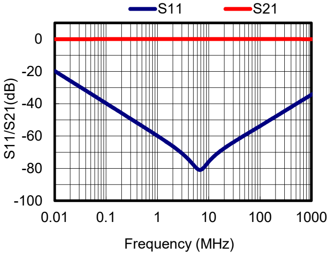
S parameters(Series)
