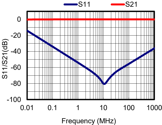
S parameters(Series)
