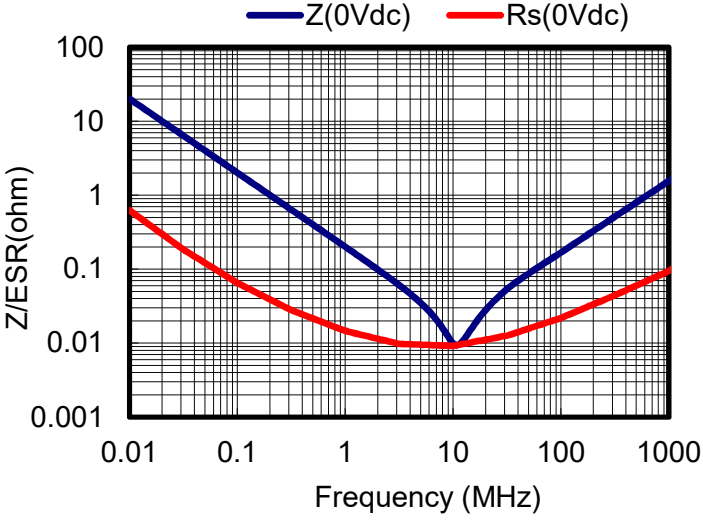
Impedance/ESR
