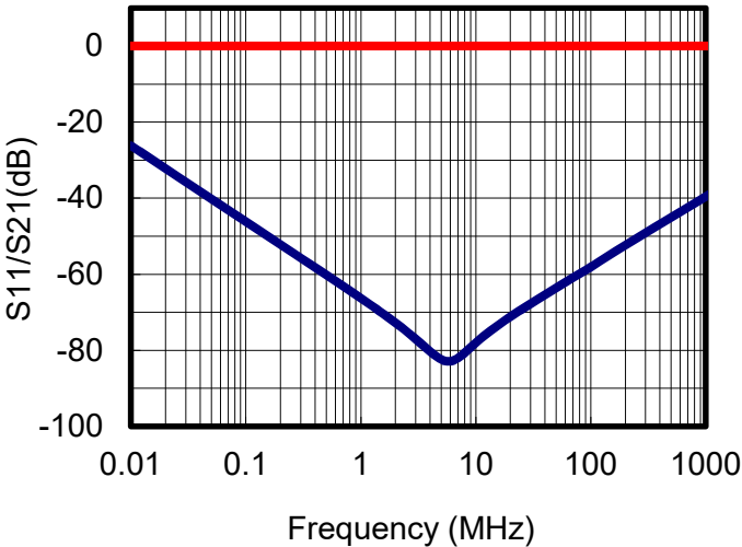
S parameters(Series)
