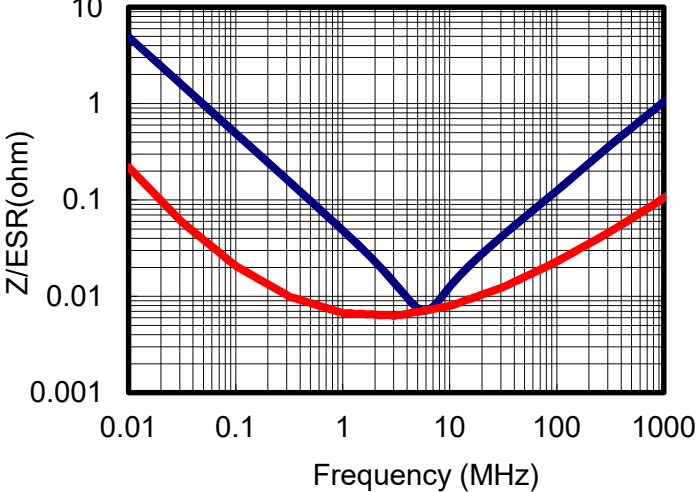
Impedance/ESR
