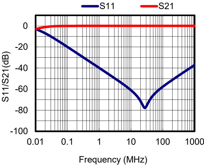
S parameters(Series)
