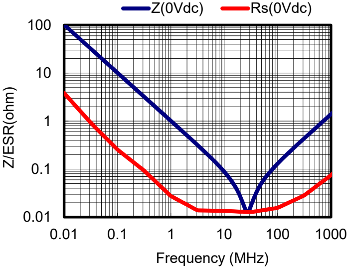
Impedance/ESR
